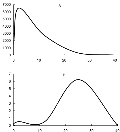
Рис. 108. Зависимость биомассы (А), плотности поселения (Б) и среднего веса экземпляра (В) Mytilus edulis от глубины. Обозначения см. на рис. 92
