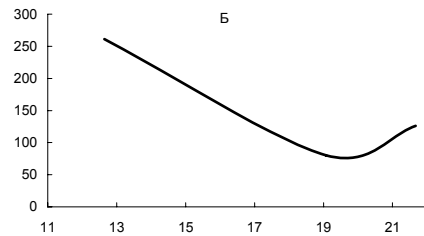
Рис. 135. Зависимость биомассы Macoma balthica от температуры (А), солёности (Б) и медианного размера частиц грунта (В). Обозначения см. на рис. 94
