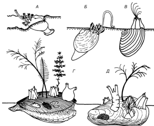
Рис. 53. Характерное размещение седвазидов на раковинах некоторых двусторчатых моллюсков. По: Наумов, Федяков, 1993. А – Portlandia arctica , Б – Macoma calcaria , В – Elliptica elliptica , Г – Clamys islandica , Д – Modiolus modiolus .
