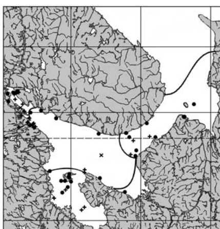
10. Musculus laevigatus
