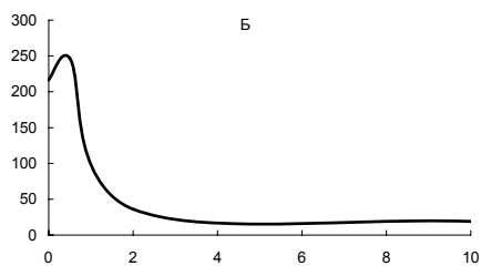
Рис. 138. Зависимость биомассы (А), плотности поселения (Б) и среднего веса экземпляра (В) Mya (Arenomya) arenaria от глубины.
