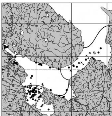
16. Heteranomia squamula
