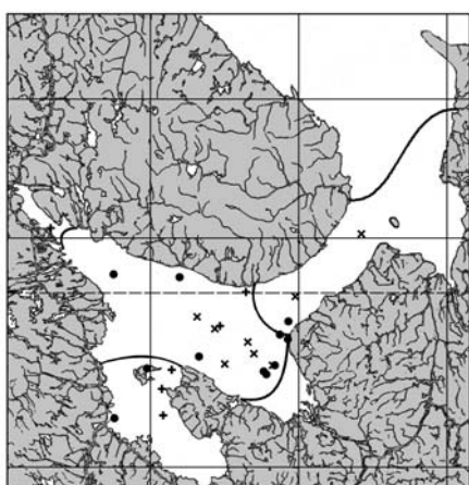
9. Musculus corrugatus
