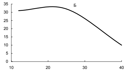
Рис. 110. Зависимость биомассы (А), плотности поселения (Б) и среднего веса экземпляра (В) Chlamys islandica от глубины. Обозначения см. на рис. 92
