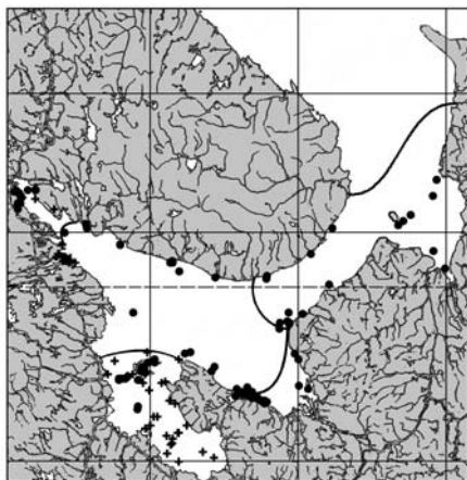
14. Mytilus edulis
