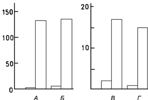
Рис. 50. Биомасса (г/м 2 , по оси ординат) Гидрозоа (А), Verruca stroemia (Б), видов рода Balanus (В) и Ascidia (Г) в сообществах, где отсутствует Modiolus modiolus (левые столбцы) и где он присутствует (правые столбцы).
