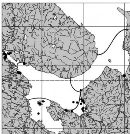
34. Macoma balthica
