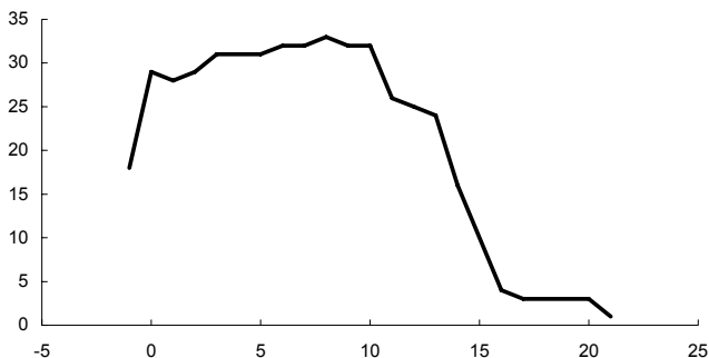
Рис. 81. Число видов беломорских двустворчатых моллюсков, встреченных при различных температурах во время гидрологического лета, по материалам БентБоМ.
