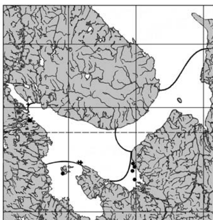
28. Axinopsida orbiculata
