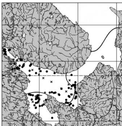
26. Thyasira gouldi
