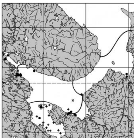
22. Tridonta borealis
