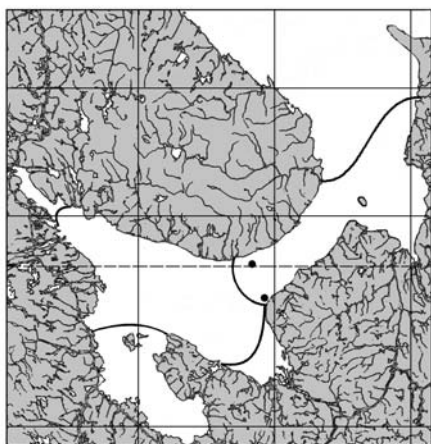
38. Lyonsiella abyssicola
