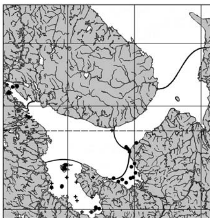
32. Serripes groenlandicus
