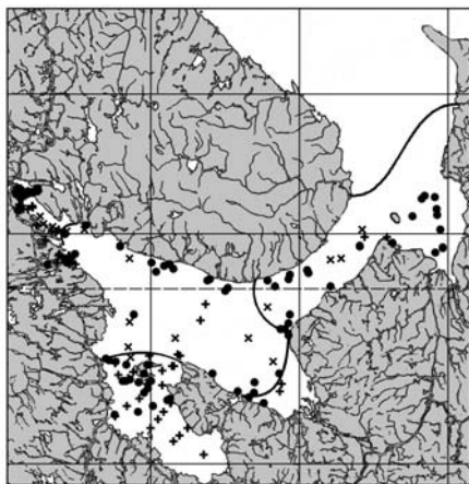
24. Hiatella spp.
