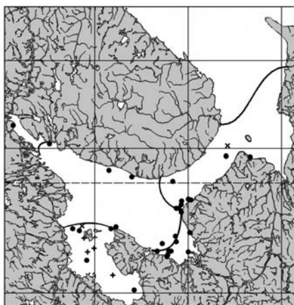
20. Thracia myopsis
