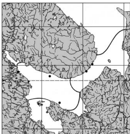
29. Turtonia minuta
