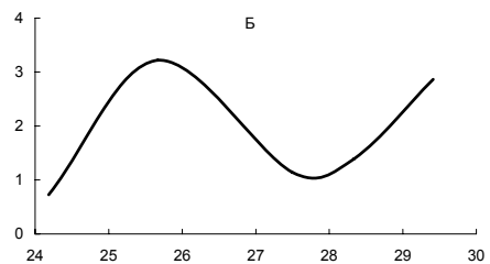
Рис. 120. Зависимость биомассы Nicania montagui от температуры (А), солёности (Б) и медианного размера частиц грунта (В).
