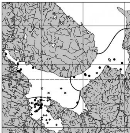
12. Modiolus modiolus
