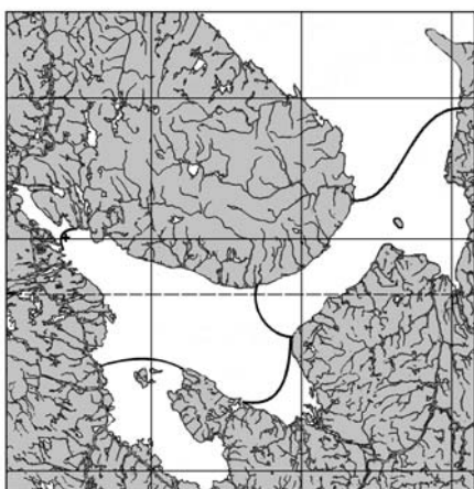
27. Thyasira equalis
