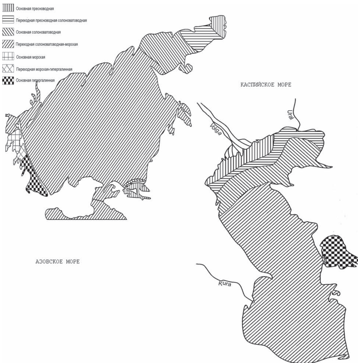
Рис. 1. Каспийское и Азовское моря и их районирование по солености (Aladin, Plotnikov, 2009).
