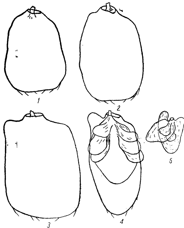
Рис. 4. Chironophora ? micronata . 1—5 — трахейные жабры. (Увел. 15).
