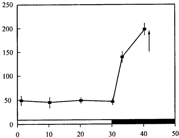
Рис. 2. Динамика размеров гермария в ходе терминации репродуктивной диапаузы у самок Harmonia sedecimnotata (второй опыт). Обозначения, как на рис. 1.
