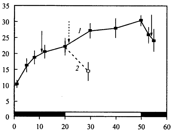
Рис. 3. Динамика сухого веса самок Harmonia sedecimnotata в ходе индукции и терминации репродуктивной диапаузы (первый опыт).
