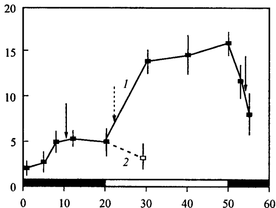
Рис. 4. Динамика весового содержания жира у самок Harmonia sedecimnotata в ходе индукции и терминации репродуктивной диапаузы (первый опыт).
