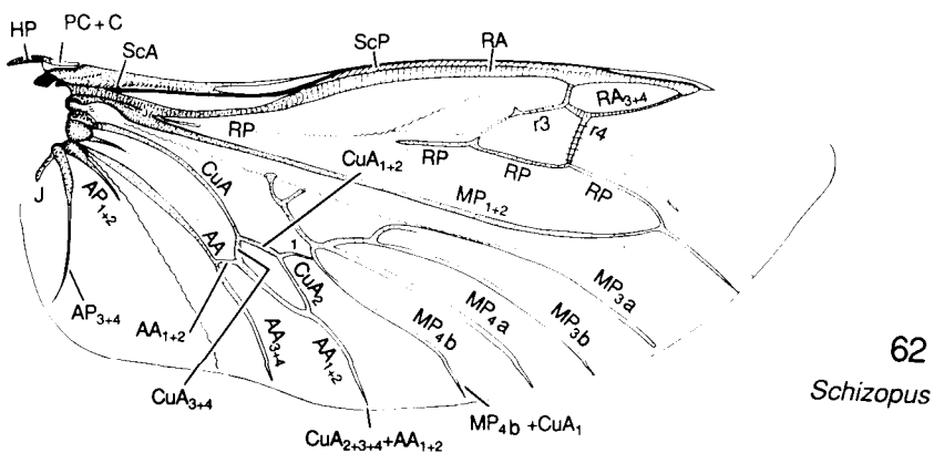
FIGS. 60-62. Elateriformia: 60, Notodascillus sublineatus Carter (Dascillidae); 61, Artematopus sp. (Artematopidae); 62, Schizopus laetus LeConte (Schizopodidae).
