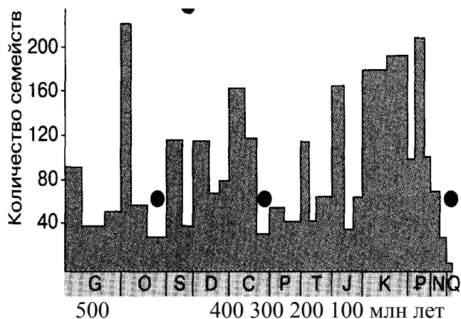
Рис. 2. Эпохи вымирания и возникновения семейств органического мира (по [9])
