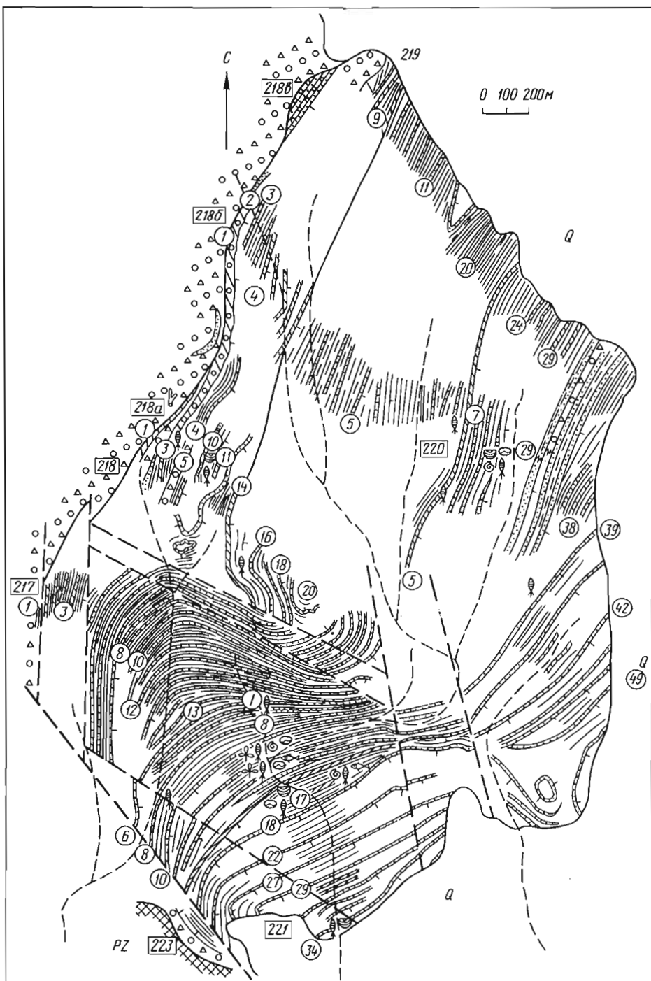
Р и с. 12. Схематическая геологическая карта местонахождения Мянгад Обозначения см. на рис. 3
