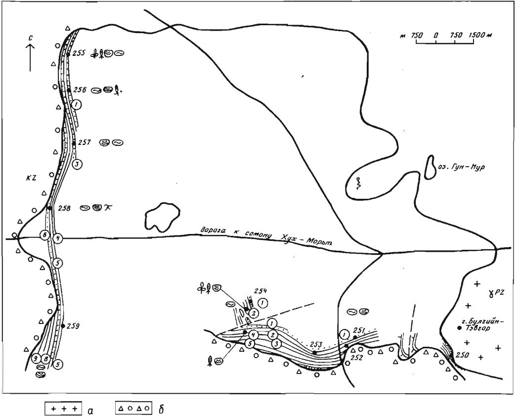
Р и с. 15. Схематическая геологическая карта местонахождения Хух-Морьт
