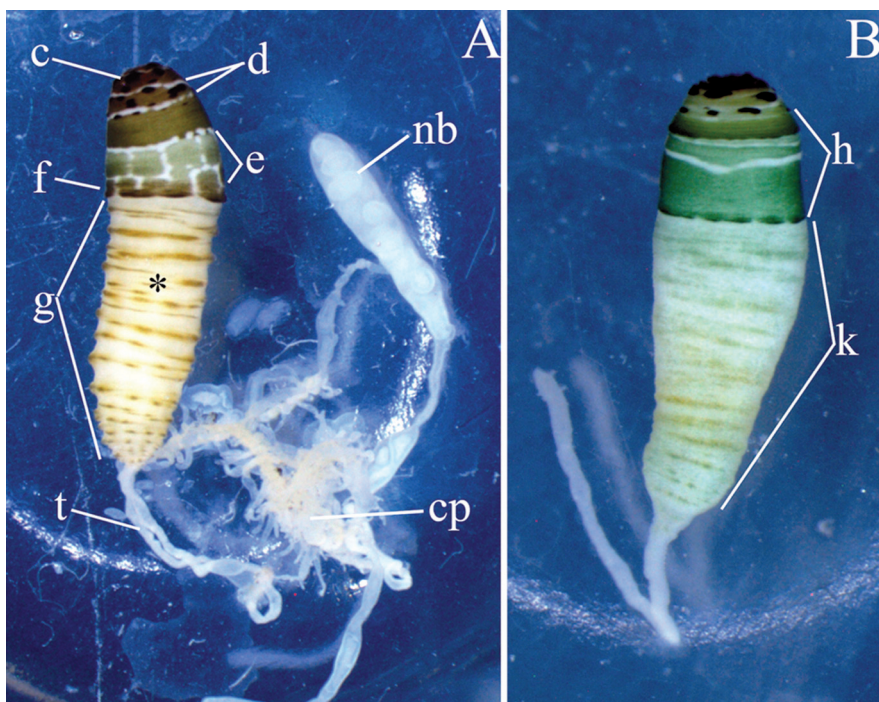
Рисунок 1. Спороцисты рода Leucochloridium : А – спороциста Leucochloridium sp., обнаруженная в моллюске Succinea putris (с – дистальный участок, окрашенный в коричневый цвет; d – поперечные белые полосы; e – участок белого цвета, на фоне которого мозаично расположены зелёные квадраты; f – прерывистая полоса коричневого цвета; g – часть отростка жёлтого цвета с характерными светло-коричневыми складками; ср – центральная часть спороцисты; nb – неокрашенный отросток; t – трубчатые участки. Звёздочка – окрашенный отросток); В – отросток L. paradoxum (h – зелёный участок; k – проксимальная часть отростка).
