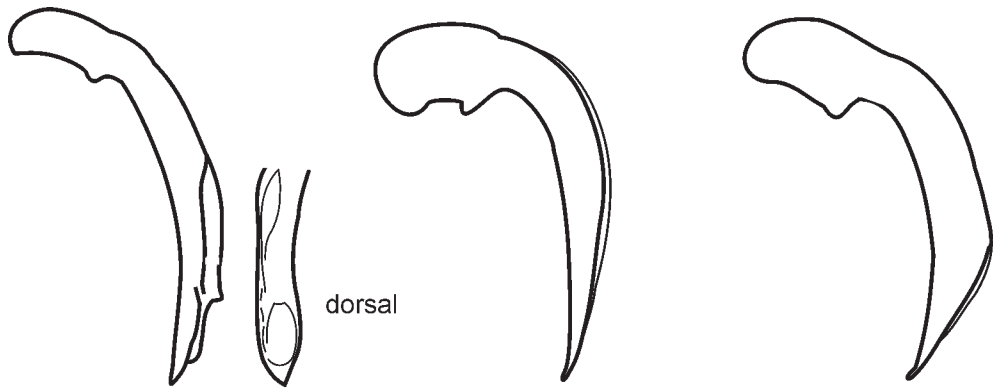
(39) Anisodactylus binotatus (40) Gaioxenus pilipalpis (41) Gnathaphanus melbournensis
