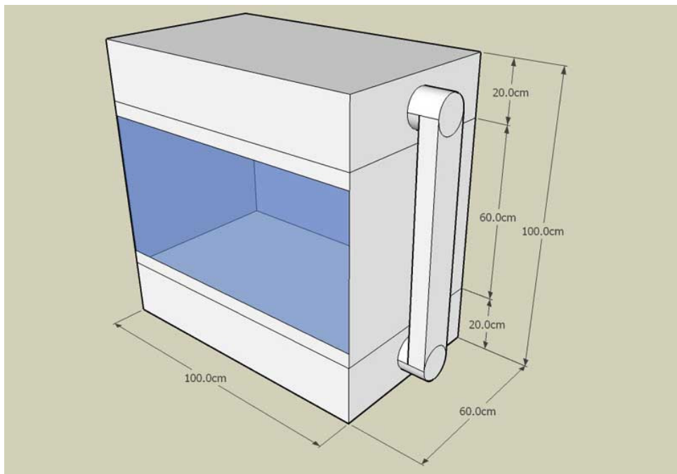
Рис. 1. Схема инкубатора для куколок тропических бабочек.
