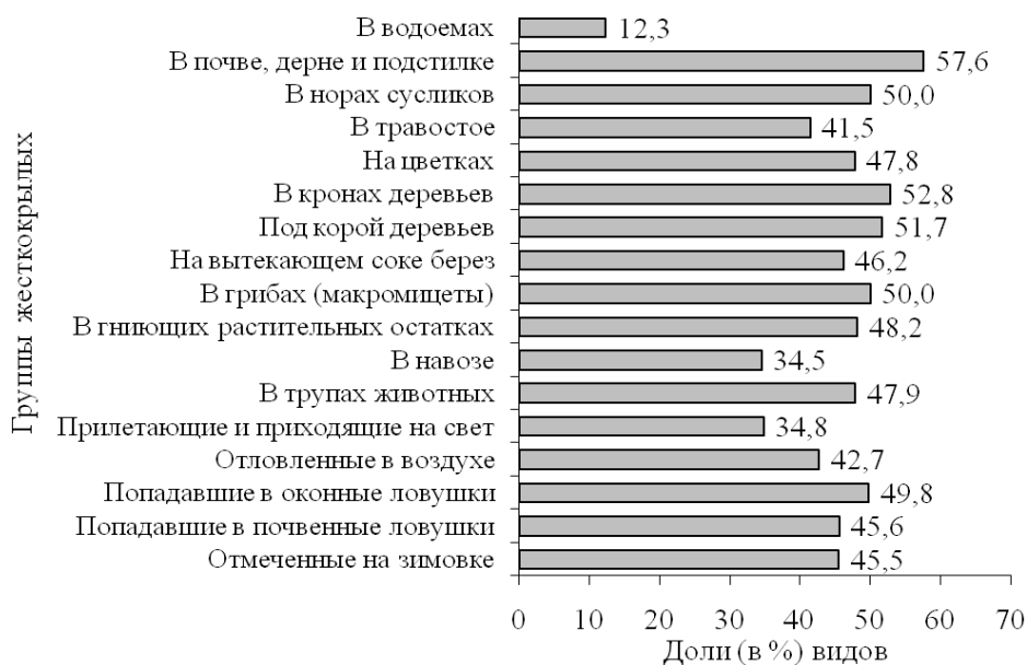
Рис. 4. Доли (в %) видов различных групп жесткокрылых, отмеченных на стенах дома
