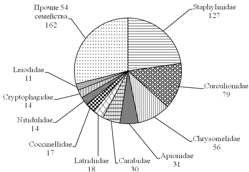
Рис. 1. Структура жесткокрылых, отмеченных на стенах дома с 1996 по 2010 гг. (указано число видов)
