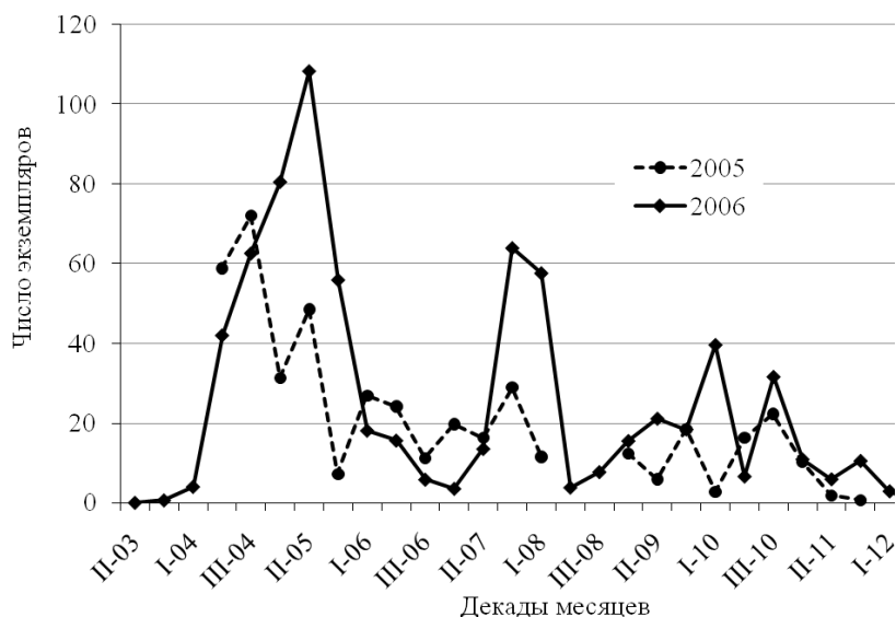
Рис. 2. Сезонная динамика численности жесткокрылых, обнаруженных на стенах дома в 2005 и 2006 гг.
