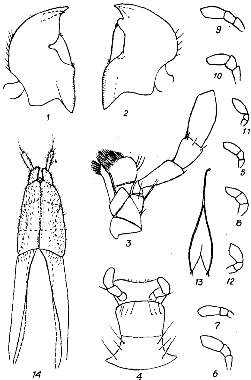
Рис. 1. Детали строения имаго Mucetophagidae:
