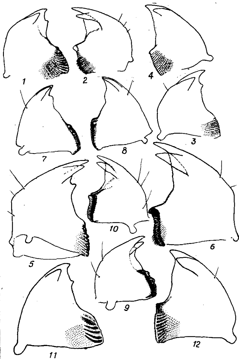
Рис.19. Мандибулы личинок видов рода Mycetophagus (вид снизу): 1, 2 - M. quadripustulatus ; 3, 4 - M. atomarius ; 5, 6 - M. grandis ; 7, 8 - M. elongatus ; 9, 10 - M. fulvicollis 11, 12 - M. incognitus
