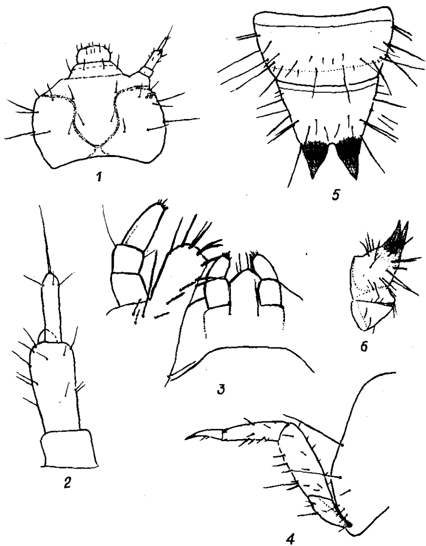
Рис. 27. Детали строения личинки Turphaea stercorea : 1 - голова; 2 - усик; 3 - максилла и нижняя губа; 4 - средняя нога; 5 - VIII-IX тергиты брюшка; 6 - IX-X сегменты брюшка (вид сбоку)
