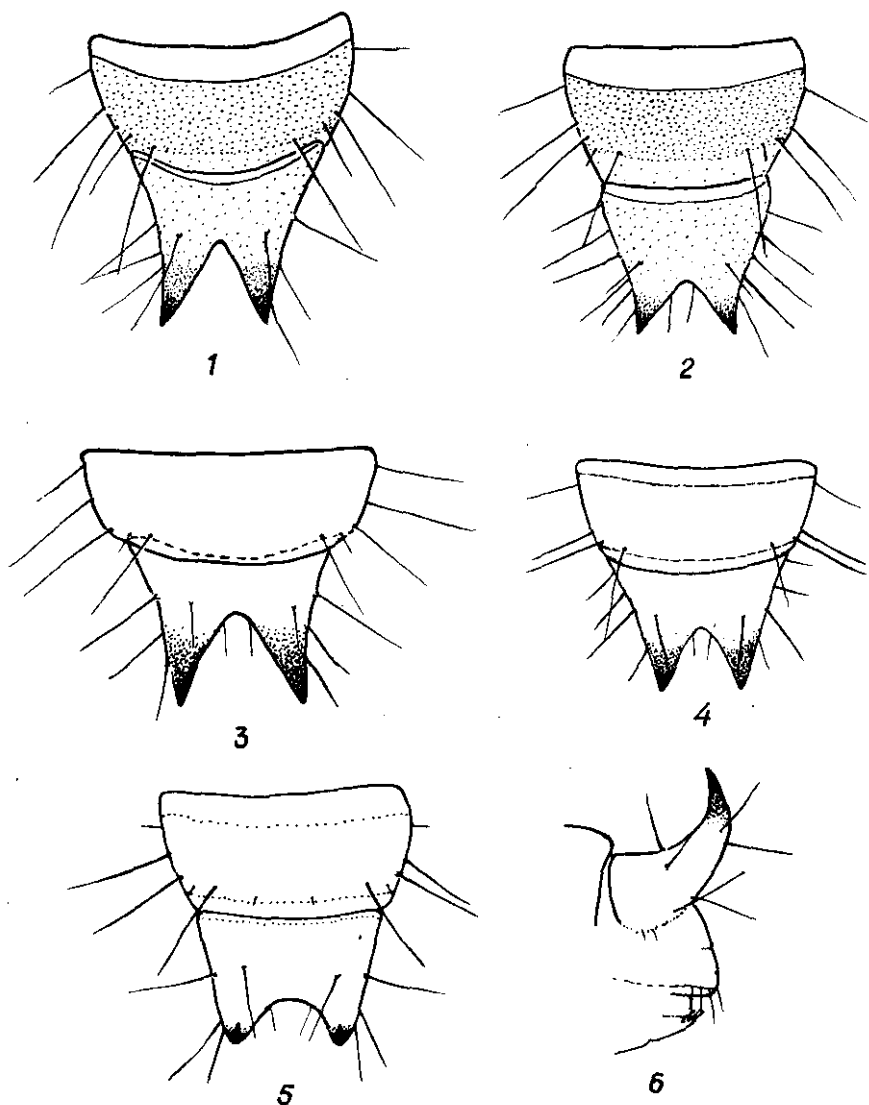
Рис. 22. Детали строения личинок видов рода Mycetophagus : 1 - VIII-IX тергиты брюшка M. quadriguttatus ; 2 - тоже, M. infulatus ; 3 - тоже, M. multipunctatus ; 4 - тоже, M. decempunctatus ; 5 - тоже, M. ciscaucasicus ; 6 - IX-X сегменты брюшка M. ciscaucasicus (вид сбоку)
