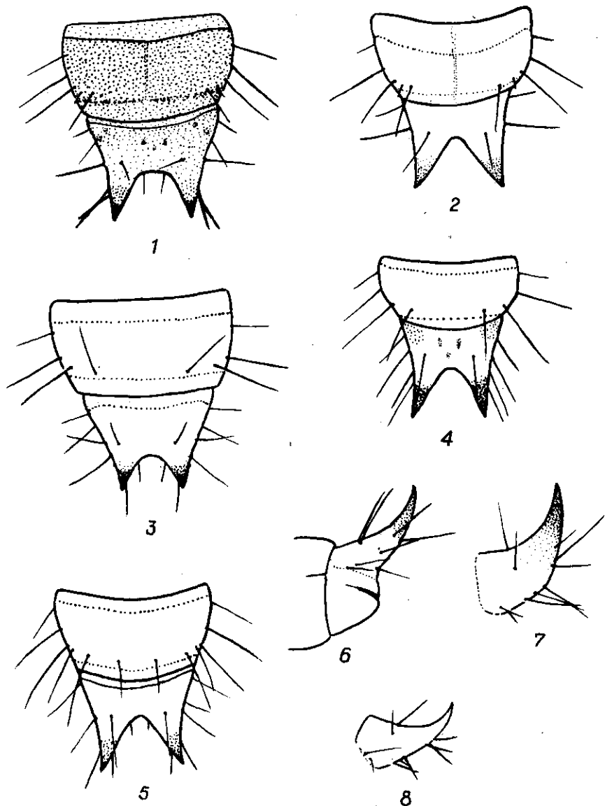
Рис. 23. Детали строения личинок видов рода Mycetophagus : 1 - VIII-IX тергиты брюшка M. grandis ; 2 - тоже, M. elongatus ; 3 - тоже, M. livshitzii ; 4 - тоже, M. tschitscherini ; 5 - тоже, M. fulvicollis ; 6 - вершинные сегменты брюшка M. tschitscherini (вид сбоку); 7 - урогомы M. antennatus (вид сбоку); 8 - тоже, M. fulvicollis (вид сбоку)
