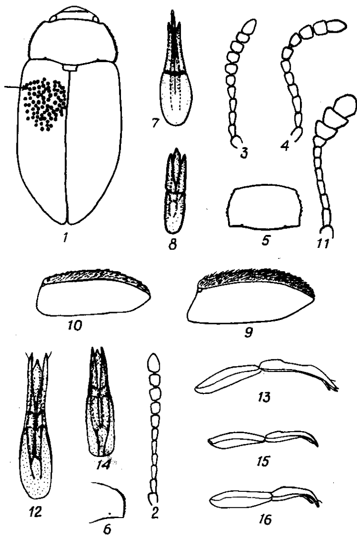
Рис. 25. Общий вид и детали строения видов рода Eulagius (1-8) и Turphaea (9-16):
