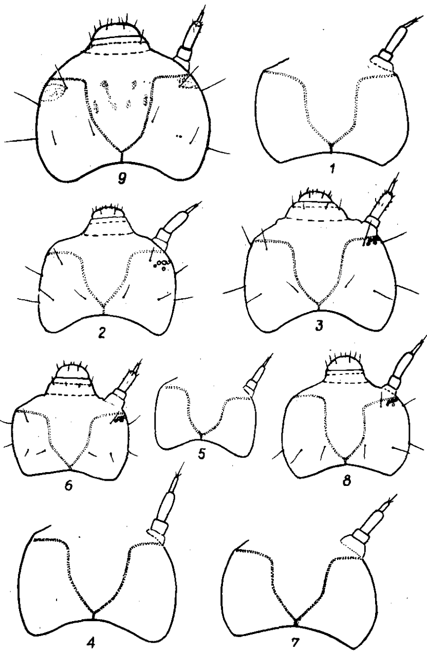
Рис. 17. Головы личинок видов рода Mycetophagus : 1 - M. quadripustulatus ; 2 - M. ancora ; 3 - M. decempunctatus ; 4 - M. antennatus ; 5 - M. piceus ; 6 - M. eiscaucasicus ; 7 - M. atomarius ; 8 - M. injulatus ; 9 - M. incognitus
