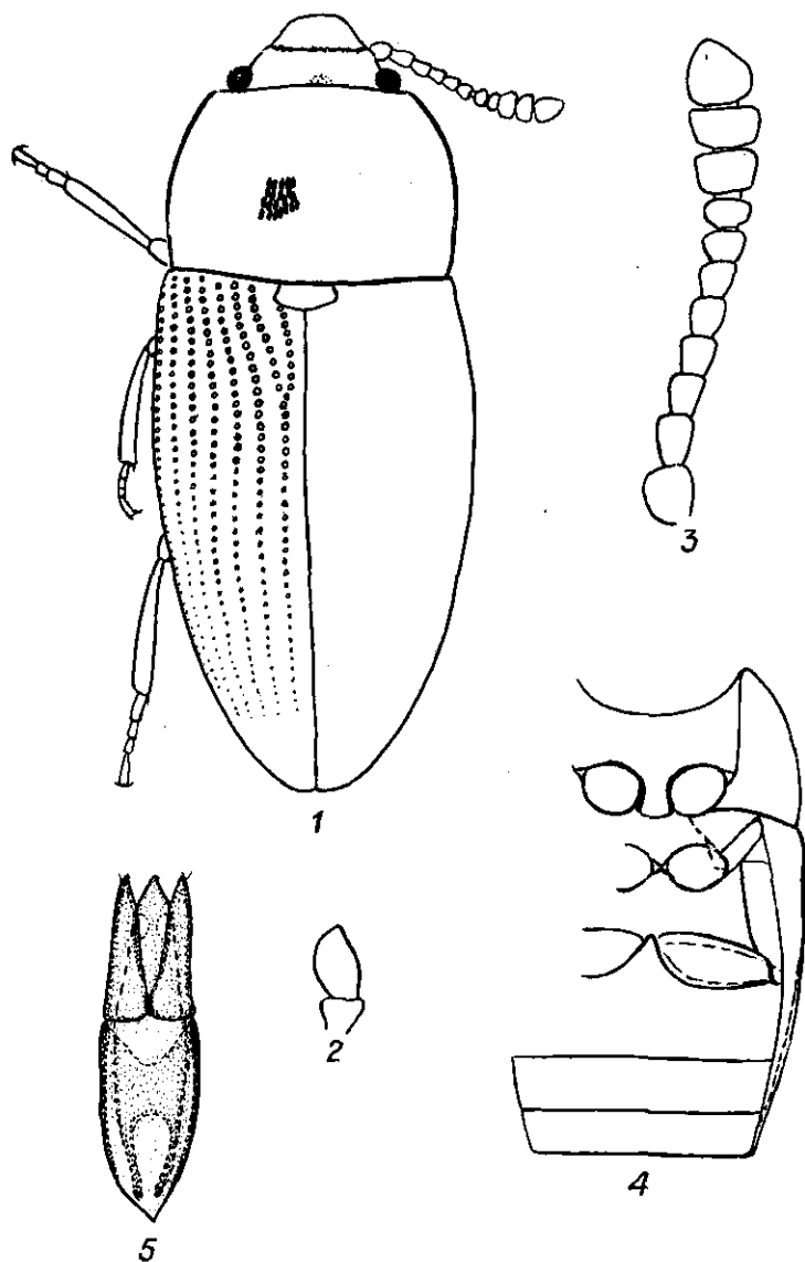
Рис. 4. Общий вид и детали строения Triphyllopsis altaicus :
