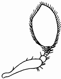
Рис. 149. Polygraphus jezoensis Niis. Усик.
