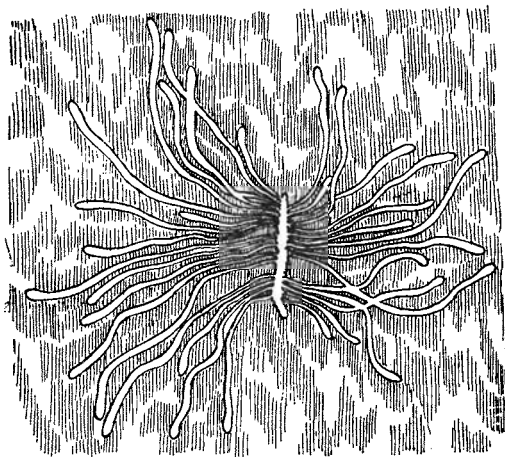
Рис. 60. Scolytus aratus Blandf. Ходы. (По Куренцову).
