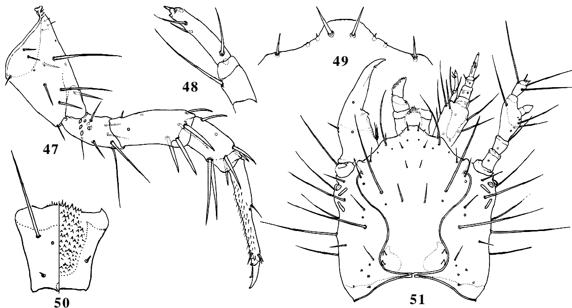
Рис. 47–51. Lebia (Lamprias) chlorocephala (Hoffmann, 1803), личинка первого возраста: 47 — нога; 48 — галея; 49 — назале; 50 — подбородок; 51 — голова (левая максилла, правые мандибула и губной щупик не показаны); 47 — спереди; 48–49, 51 — сверху; 50 — слева — сверху, справа — снизу.
