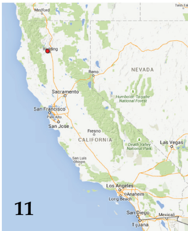
Maps 9–12. County-level distribution of Sonoma spp. 9) S. chandleri . 10) S. cobra . 11) S. colberti . 12) S. conifera .
