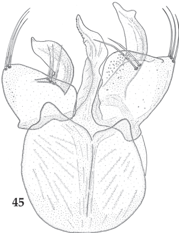
Figures 43–46. Aedeagi of Sonoma spp. 43) S. agitator new species. 44) S. rubida Casey. 45) S. humilis Marsh and Schuster. 46) S. konkoworum Chandler. Right side of figures is anatomical left.
