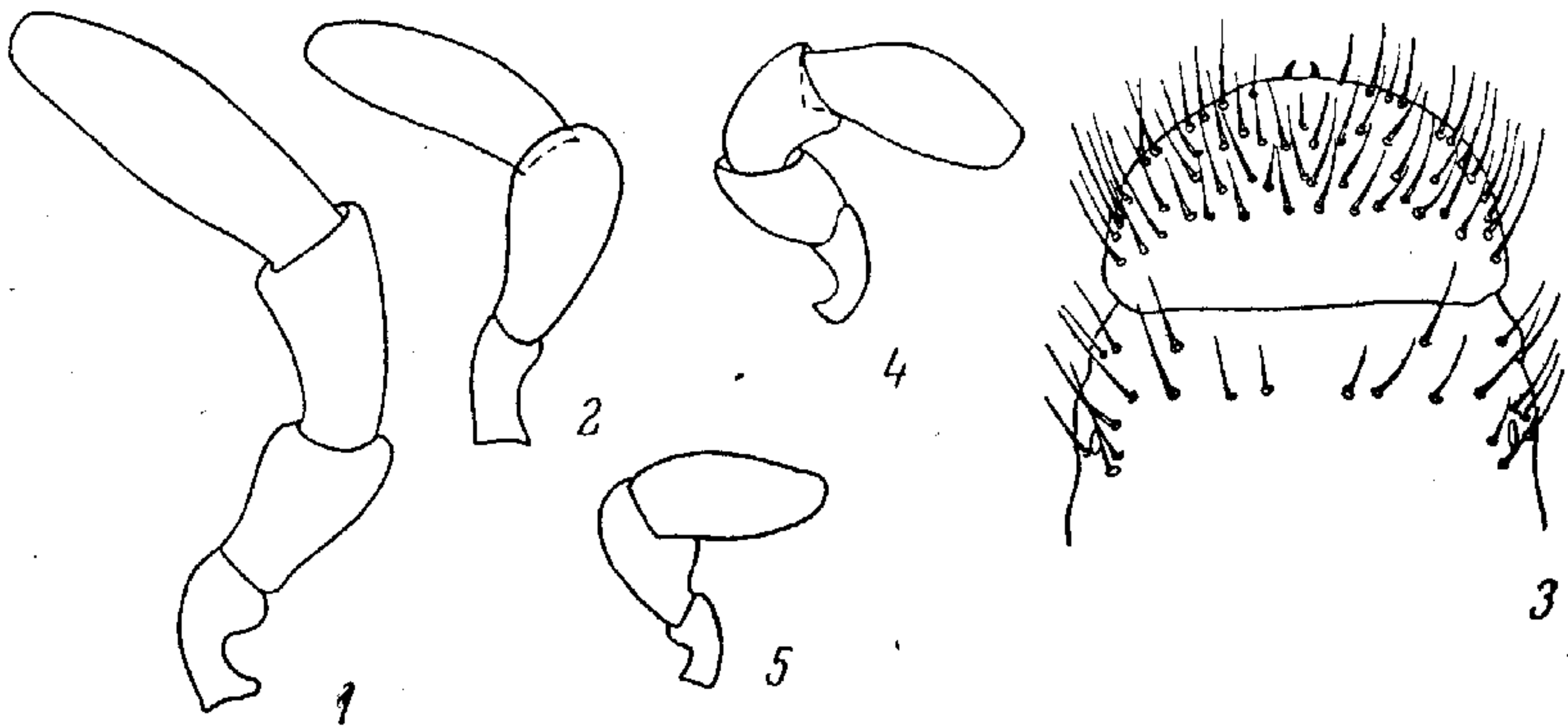
Рис. 1—5. Parmena Latr.
